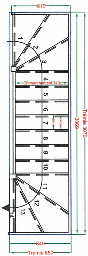
Escalier de 2860 mm de hauteur
